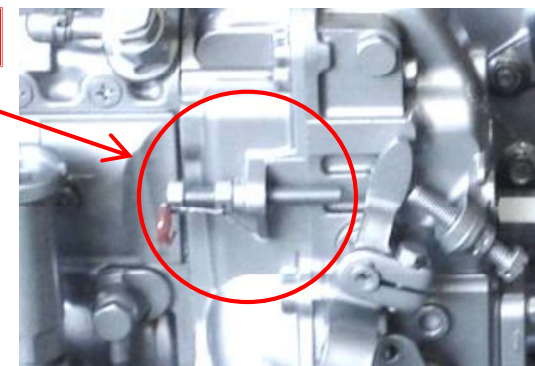
封印状況(制限装置カラー写真)
