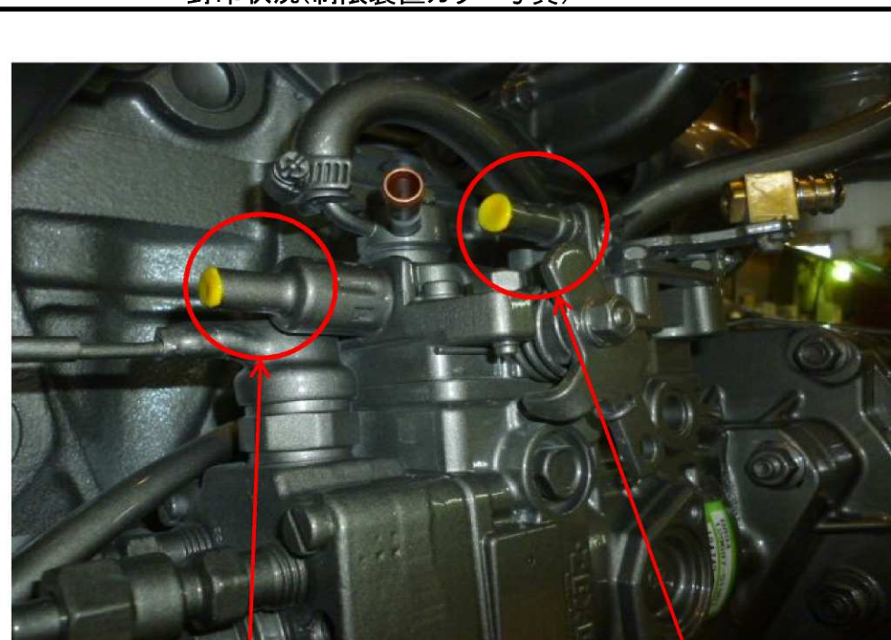
封印状況(制限装置カラー写真)
